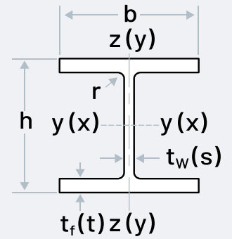
Statische Kennwerte / Section properties / Valeurs statiques
